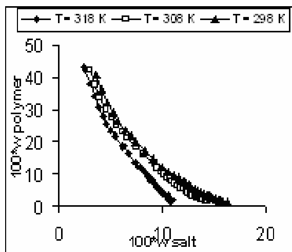
Рис. 2. Влияние температуры на область гетерогенности в системе ПЭГ-Na 2 C 4 H 4 O 6 -H 2 O
