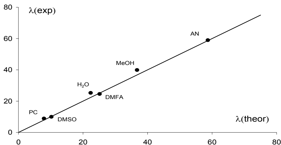
Рис. 1 Сравнение рассчитанных \lambda(\text{theor}) и экспериментальных \lambda(\text{exp}) предельных молярных электрических проводимостей \text{K18C6}^+ в различных растворителях при 25 °С. Линия соответствует \lambda(\text{theor}) = \lambda(\text{exp}) .
