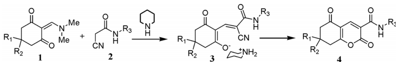
Рис. 1. Схема синтеза производных 2,5-диоксо-5,6,7,8-тетрагидро-2Н-хромена
