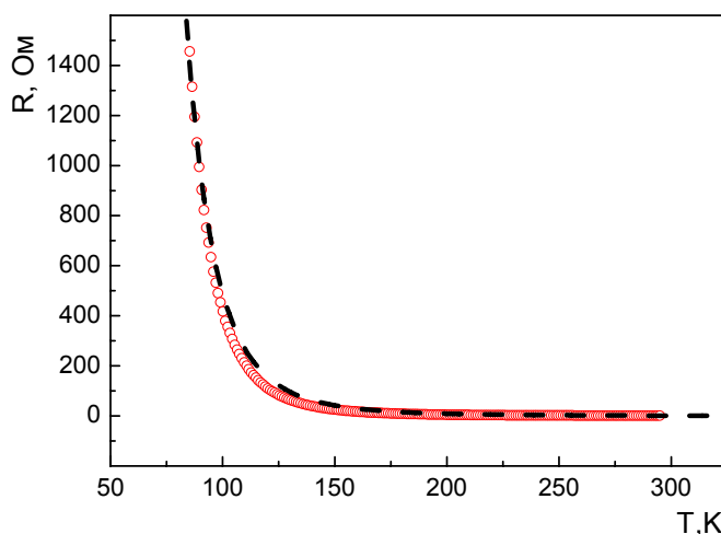
Рис. 3. Температурная зависимость сопротивления соли (TMTTF)_2WO_3S .
