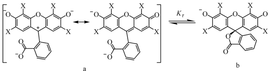
Рис. 1. Флуоресцеин (I) X = H; Эозин (II) X = Br; 2,4,5,7-тетранитрофлуоресцеин (III) X = NO 2 ; а – хиноидная структура; б – лактонная структура.
