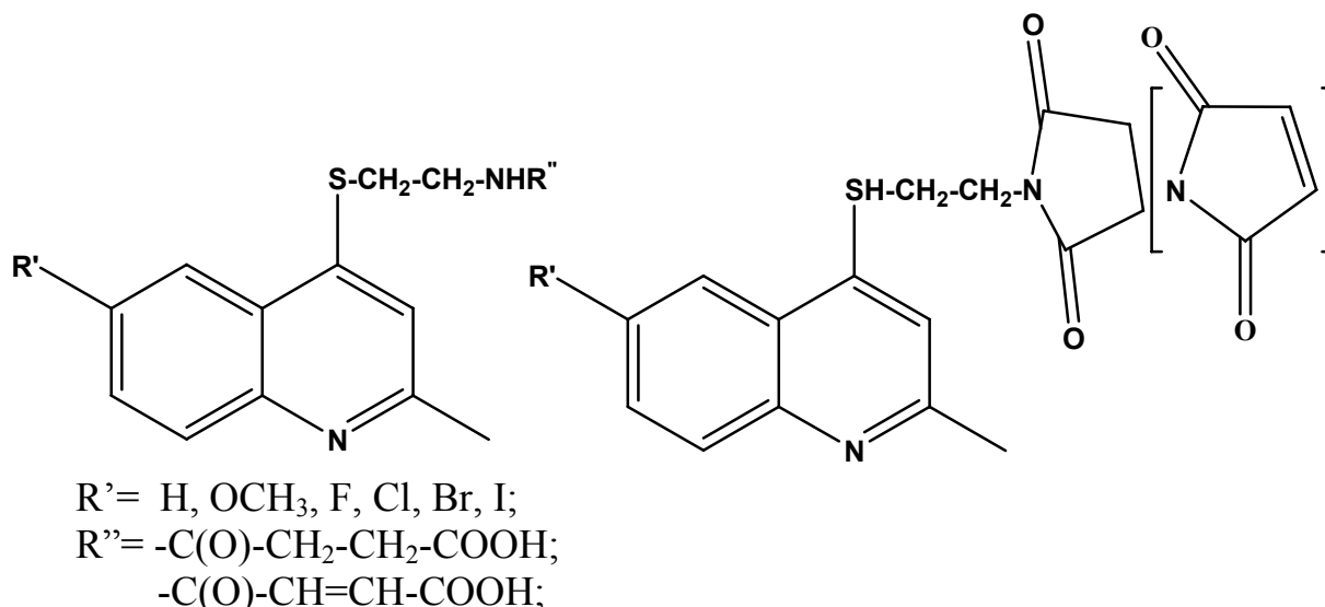
Рис. 1. Похідні S-(2-метилхінолін-4-іл)цистеамідів(імідів) дикарбонових кислот
